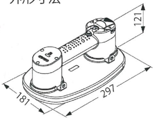
外形寸法
