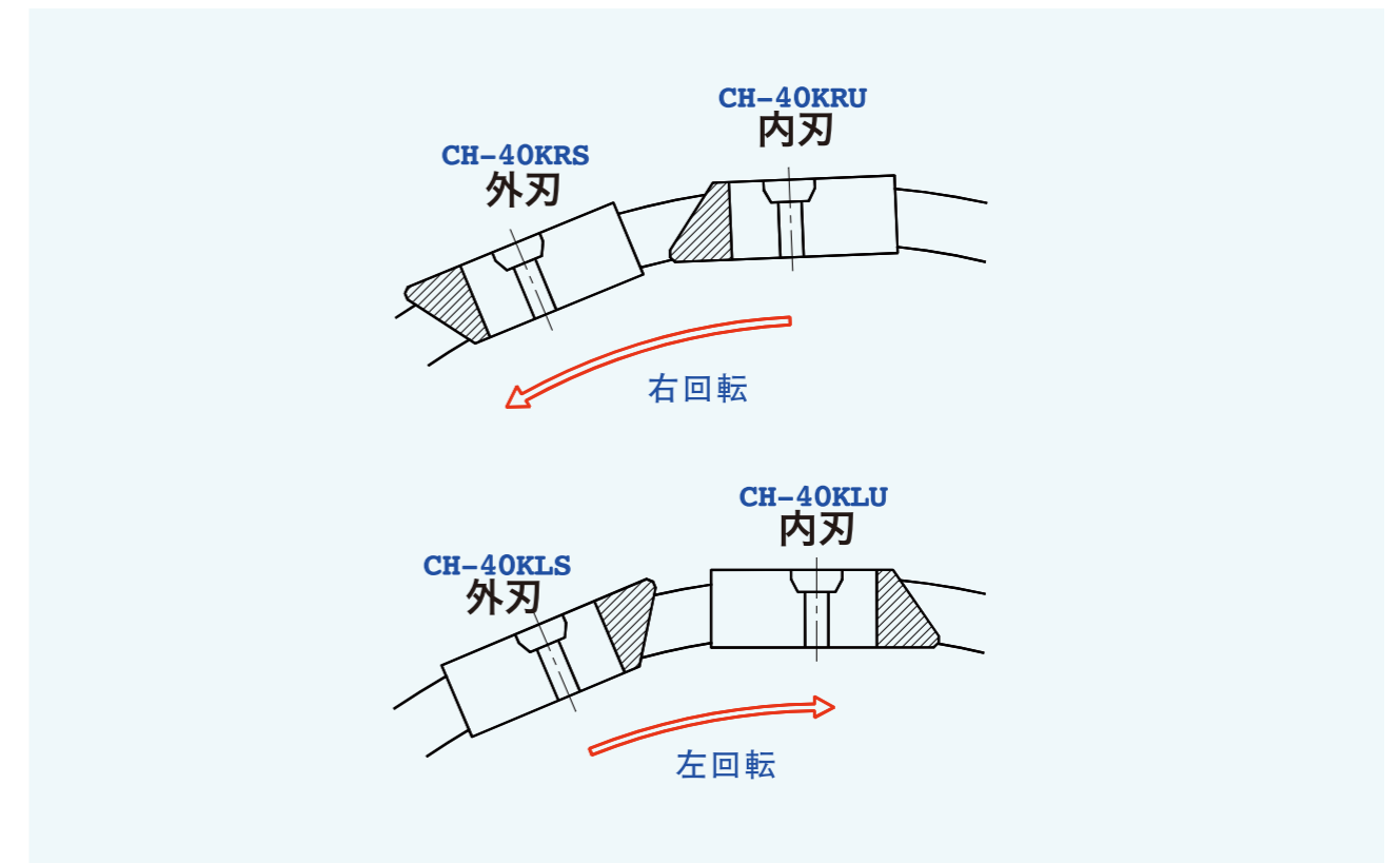
ケーシングの回転方向と外刃と内刃の関係
